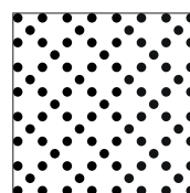
Acoustiroc® ASTRAL 17% Ø2,5 (rond, régulière) \alpha_w = 0,95 NRC : 0,90
