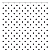
Acoustiroc® INFINITY 11% Ø1,5 (rond, régulière) \alpha_w = 0,95 NRC : 0,90
