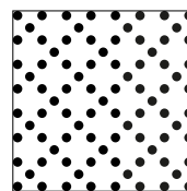
Acoustiroc® ASTRAL 17% Ø2,5 (rond, régulière) \alpha_w = 0,95 NRC : 0,90
